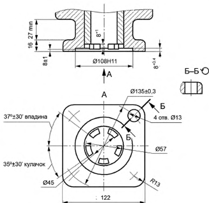
Рисунок А.9 — Присоединение привода типа Б
