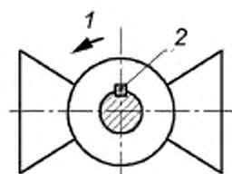
Рисунок 12 — Положение одной шпонки на шпинделе закрытой арматуры
