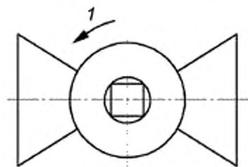
Рисунок 16 — Положение параллельной квадратной головки на закрытой арматуре
