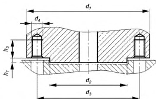
Рисунок 2 — Присоединения типов F03—F100
