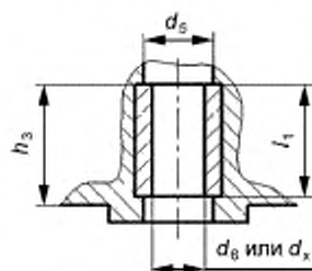
Рисунок 4 — Ведущая подвижная деталь группы А
