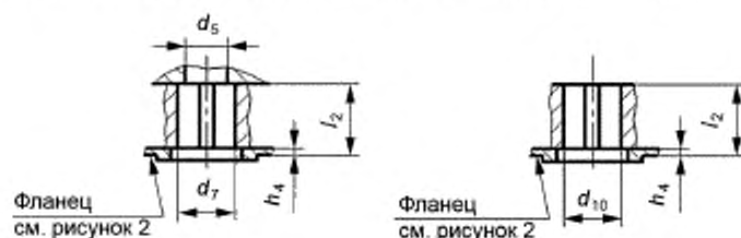
Рисунок 6 — Ведущие подвижные детали группы В
