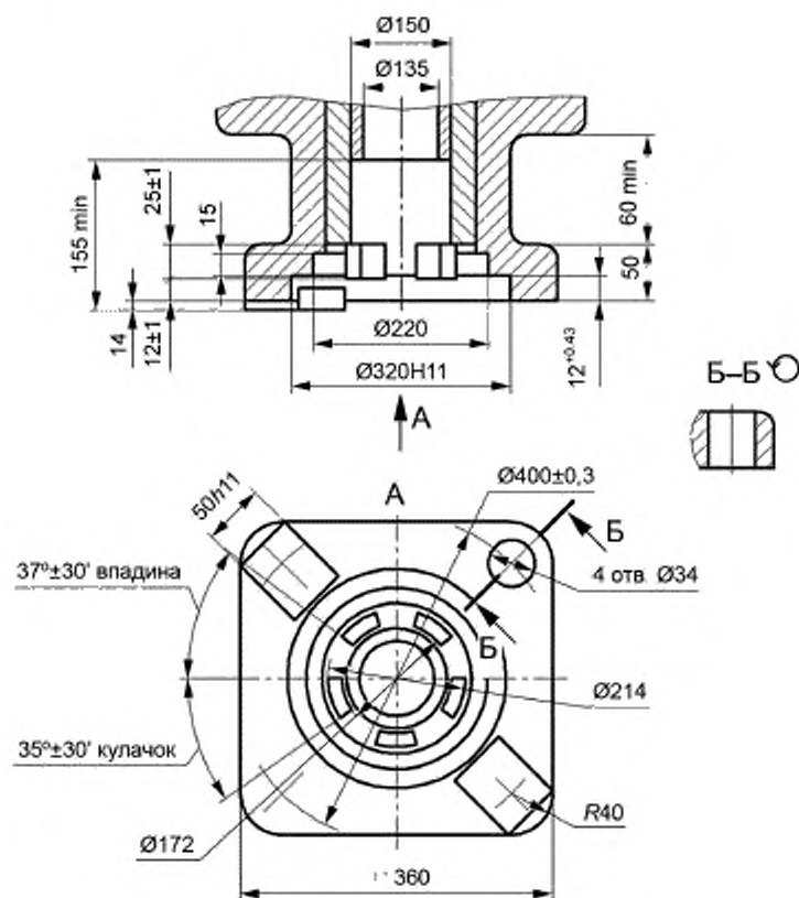
Рисунок А.13 — Присоединение привода типа Д
