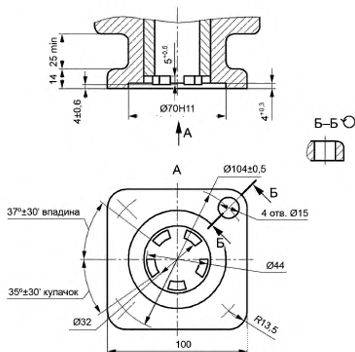
Рисунок А.7 — Присоединение привода типа АК
