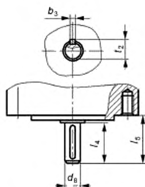
Рисунок 9 — Ведущие подвижные детали группы D
