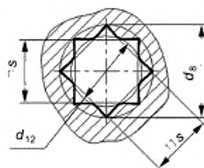
Рисунок 21 — Соединения через восьмигранник
