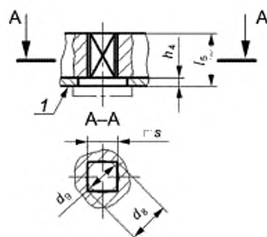
Рисунок 14 — Соединение с параллельной квадратной головкой
