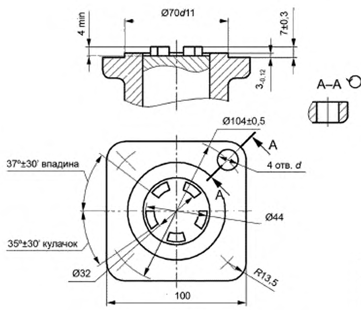
Рисунок А.8 — Ответное присоединение трубопроводной арматуры типа АК
