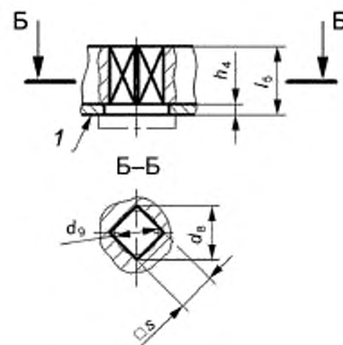
Рисунок 15 — Соединение с диагональной квадратной головкой
