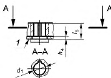
Рисунок 11 — Передача крутящего момента через шпонку
