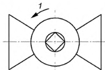
Рисунок 17 — Положение диагональной квадратной головки на закрытой арматуре
