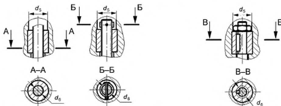
Рисунок 4 — Ведущая подвижная деталь группы А
