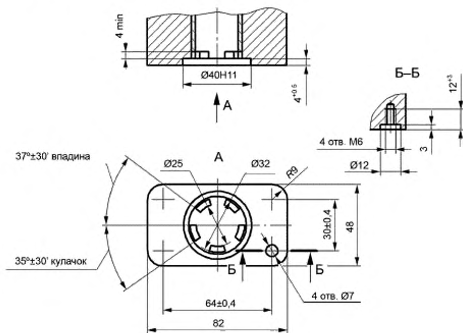
Рисунок А.3 — Присоединение привода типа МК
