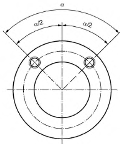
Рисунок 3 — Расположение отверстий для типов присоединений F03—F100
