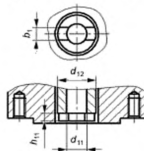
Рисунок 8 — Ведущие подвижные детали группы С
