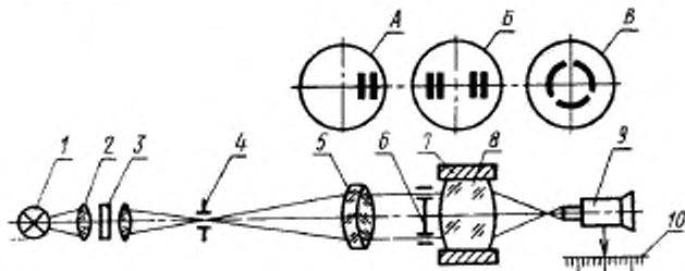
1 — источник света; 2 — конденсор; 3 — сменный интерференционный светофильтр; 4 — раздвижная щель; 5 — коллиматор; 6 — диафрагма: А — с одной парой щелей, Б — с двумя парами щелей, В — кольцевая; 7 — объективодержатель; 8 — испытуемый объектив; 9 — микроскоп
