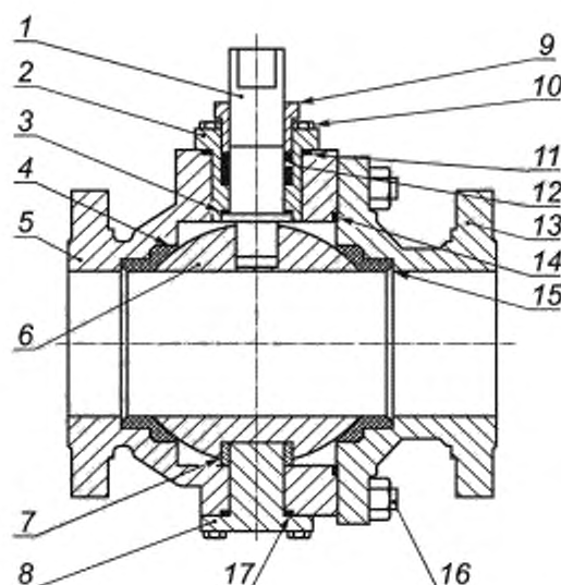
1 — шпindel; 2 — крышка; 3 — упорное кольцо; 4 — седло; 5 — корпус крана; 6 — шаровая пробка; 7 — подшипник опоры; 8 — опора шара; 9 — втулка сальника; 10 — крепеж крышки; 11 — уплотнение крышки; 12 — уплотнение шпинделя (сальниковая набивка); 13 — фланец; 14 — уплотнение корпуса; 15 — пружина седла; 16 — крепеж корпуса; 17 — уплотнение опоры
