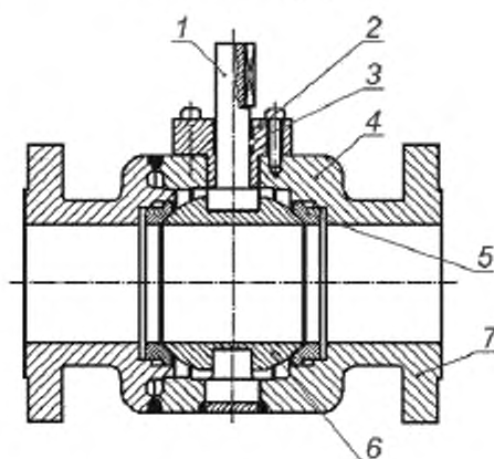
1 — шпindel; 2 — крышка; 3 — уплотнение шпинделя (сальниковая набивка); 4 — сварной корпус крана; 5 — седло; 6 — шаровая пробка; 7 — фланец корпуса
