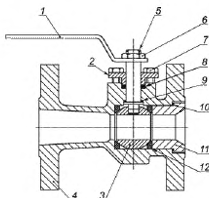
1 — рукоятка; 2 — втулка сальника; 3 — шаровая пробка; 4 — корпус; 5 — шпindelь; 6 — гайка, — крепеж втулки сальника; 8 — сальник; 9 — упорное кольцо; 10 — уплотнение корпуса; 11 — корпусная втулка; 12 — седло
