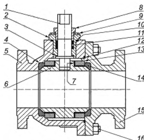
1 — шпindelь; 2 — крышка; 3 — упорное кольцо; 4 — седло; 5 — корпус крана; 6 — шаровая пробка; 7 — радиальный подшипник опоры (подшипник скольжения); 8 — втулка сальника; 9 — крепеж крышки; 10 — уплотнение крышки; 11 — уплотнение шпинделя (сальниковая набивка); 12 — уплотнение корпуса; 13 — плоская опора; 14 — торцевой подшипник опоры (подшипник скольжения); 15 — фланец; 16 — крепеж корпуса
