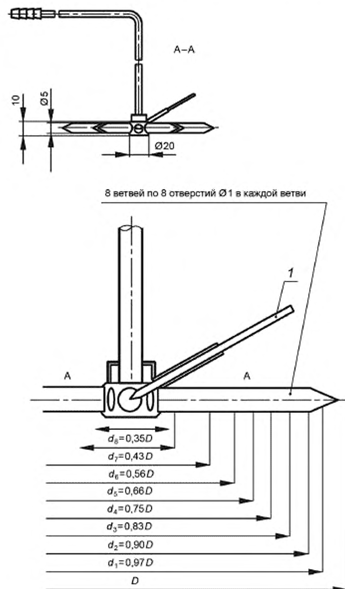
Рисунок 101 — Пробоотборник для отбора проб и измерения температуры продуктов сгорания для дымохода диаметром более 100 мм
