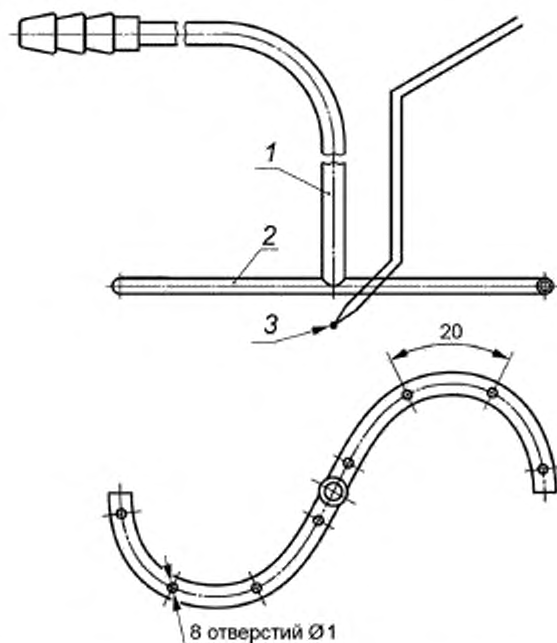
1 — медная трубка диаметром 8 мм; 2 — медная трубка диаметром 4 мм; 3 — термопара
