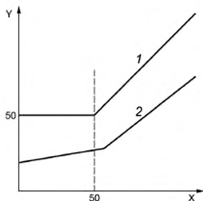
1 — граница чувствительности. см. 3.105; 2 — настройка чувствительности см. 3.106 X — поток газа, \text{м}^3/\text{ч} ; Y — установленная скорость утечки, \text{дм}^3/\text{ч}
