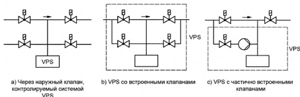
Рисунок 2 — Примеры конфигурации системы VPS
