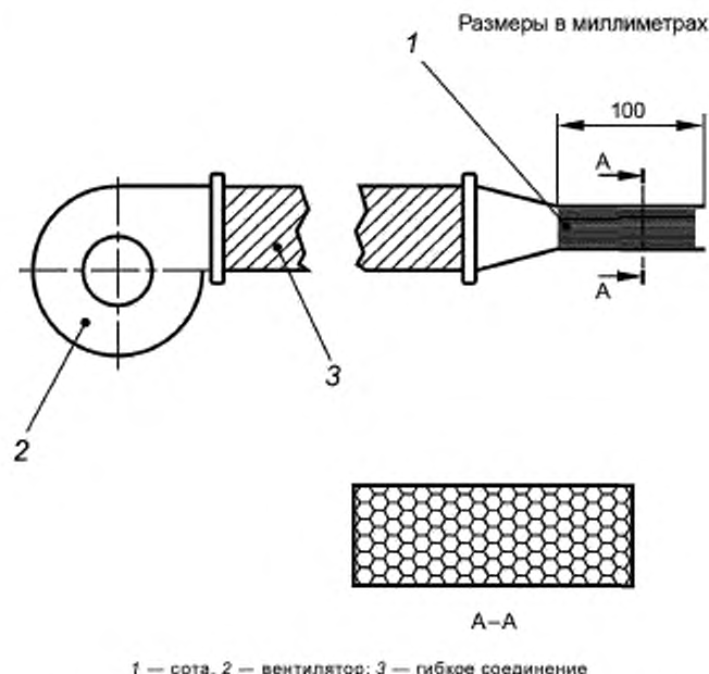
Рисунок 2 — Устройство для испытания на ветровую нагрузку
