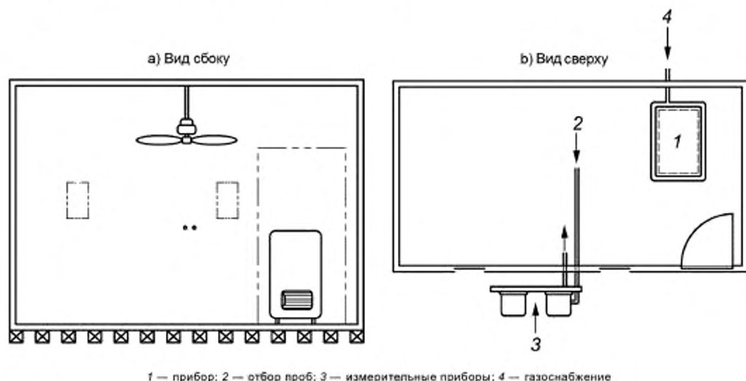
Рисунок F.1 — Пример климатической камеры
