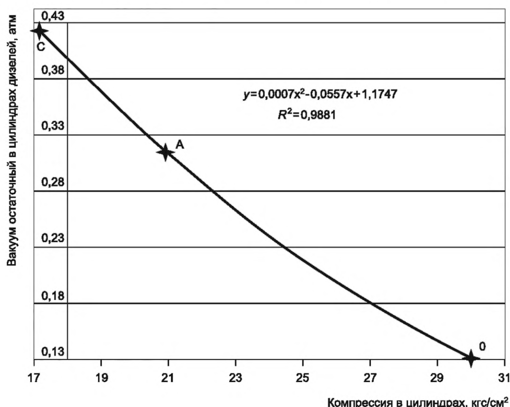
Рисунок Е.1 — График оценки остаточного ресурса цилиндров тракторных и комбайновых двигателей по взаимосвязи остаточного вакуума и компрессии в цилиндрах
