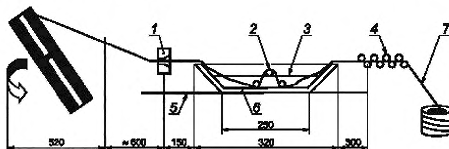
1 — фильера диаметром 1,1 мм; 2 — плоские направляющие стержни; 3 — уровень смолы; 4 — натяжители; 5 — регулируемая опора; 6 — пропиточная ванна (с регулируемой температурой); 7 — ролинг
