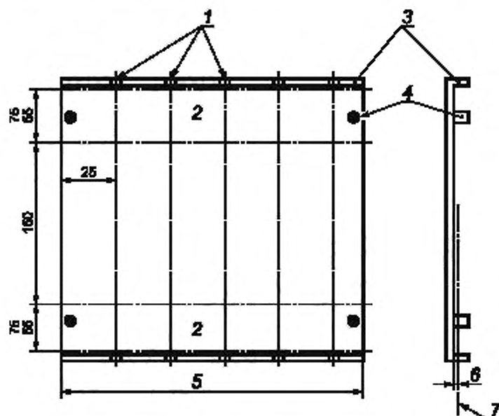
1 — прорезы для ровингов; 2 — полосы картона или композита; 3 — стенка; 4 — проставки; 5 — размеры зависят от количества образцов; 6 — толщина картона или композита; 7 — уровень нижнего края надразов
