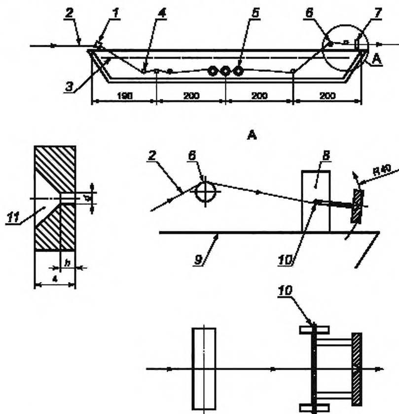
1 — подающий направляющий ролик; 2 — ровинг; 3 — уровень смолы; 4 — плоские направляющие стержни; 5 — рельефные направляющие стержни; 6 — приемный направляющий ролик; 7, 11 — фильера; 8 — держатель фильеры; 9 — ванна для пропитки; 10 — вращающийся шпиндель фильеры; d — диаметр отверстия фильеры; h — высота отверстия фильеры
