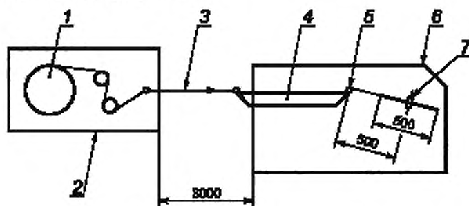
1 — бобина ровинга или паковка; 2 — шпулярник, оборудованный натяжителями; 3 — ровинг; 4 — ванна для пропитки; 5 — фильера; 6 — намоточный станок; 7 — оправка
