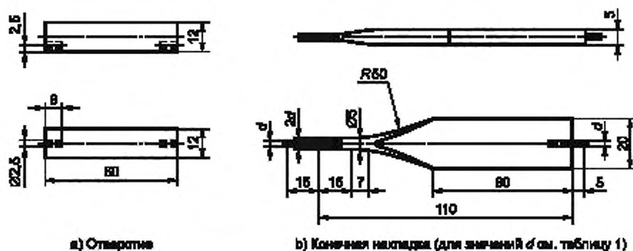
Рисунок 6 — Алюминиевый шаблон
