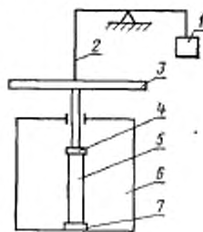
1—противовес; 2—проволока; 3—инерционная лента; 4—верхний подвижный зажим; 5—образец; 6—термостатирующая камера; 7—нижний неподвижный зажим
