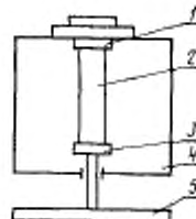
1—верхний неподвижный зажим; 2—образец; 3—нижний подвижный зажим; 4—термостатирующая камера; 5—инерционная деталь
