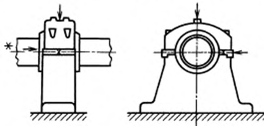
Положение точек измерения вибрации для машин с высотой оси вращения более 400 мм со стоячковыми подшипниками (применимо для обеих сторон машины)
