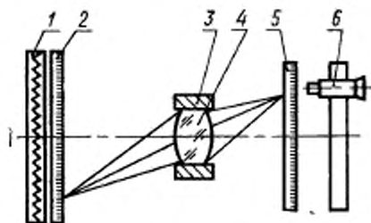
1—осветитель шкалы; 2—шкала в предметной плоскости; 3—объективодержатель; 4—испытуемый объектив; 5—шкала в плоскости изображения; 6—микроскоп.
