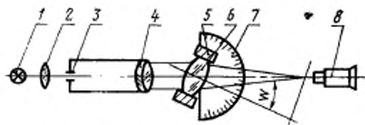
1—источник света; 2—конденсор; 3—раздвижная щель; 4—коллиматор; 5—объективодержатель; 6—испытуемый объектив; 7—шкала отсчета угловых перемещений объектива; 8—микроскоп.
