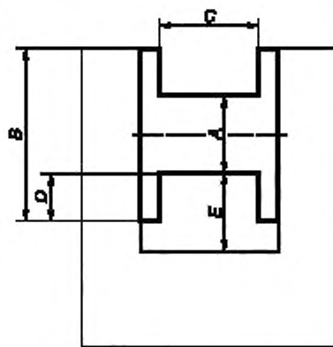
Рисунок 1 — Схема к определению основных размеров барабана лебедки*
