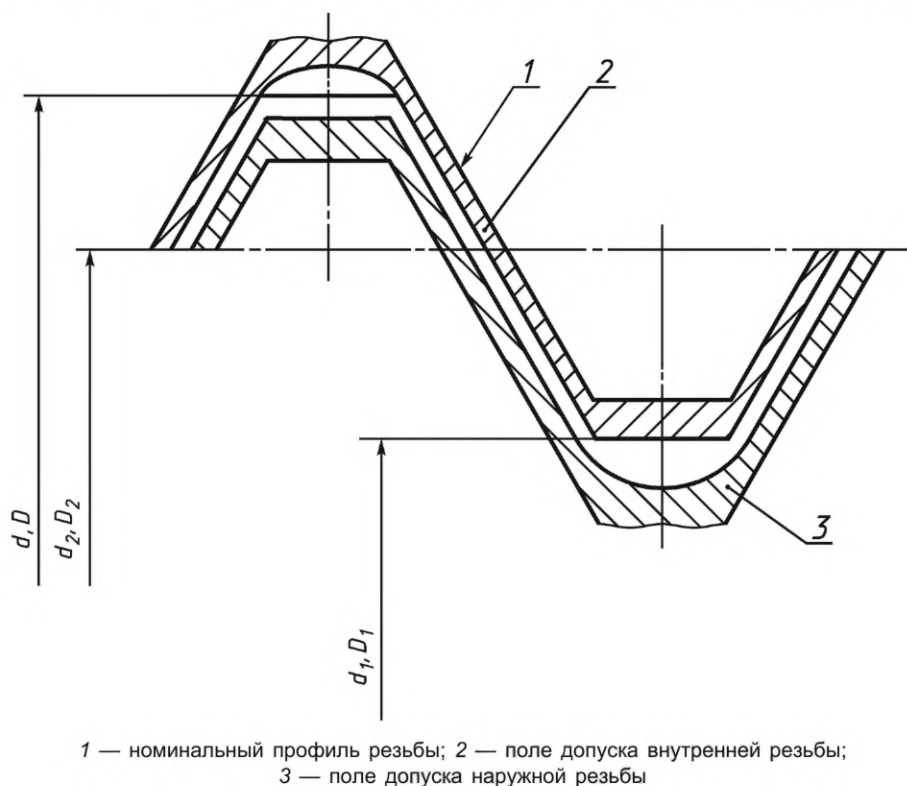
Рисунок 10 — Расположение полей допусков резьбы
