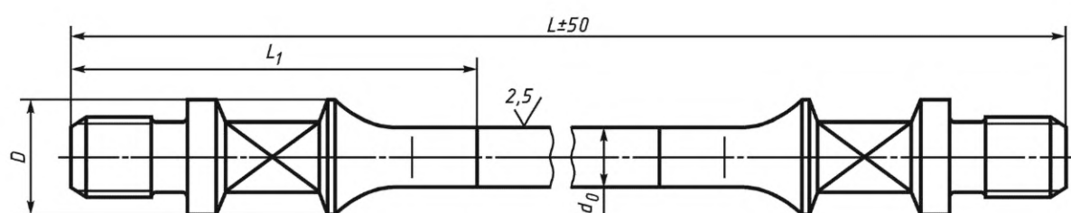
б — металлическая штанга с приваренными головками (ШНП)
