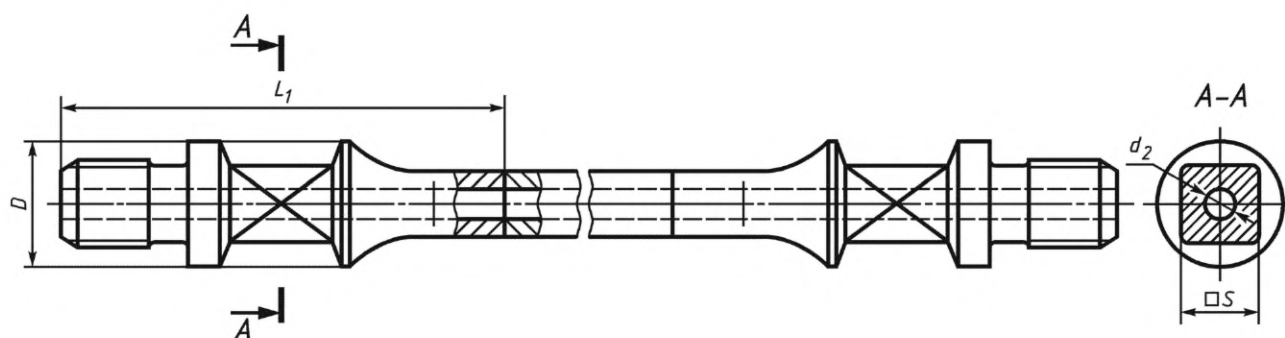
6 — металлическая полая штанга с приваренными головками (ШНПП)
