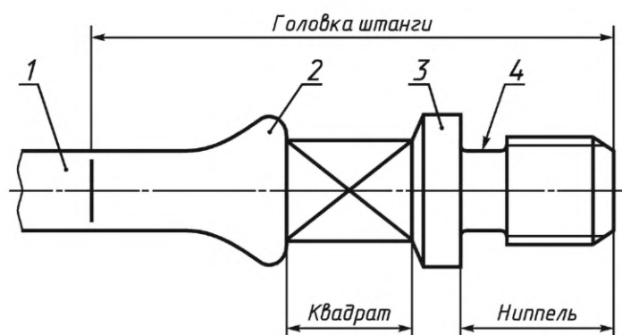
1 — тело штанги; 2 — подэлеваторный бурт; 3 — упорный бурт; 4 — резьбовая канавка
