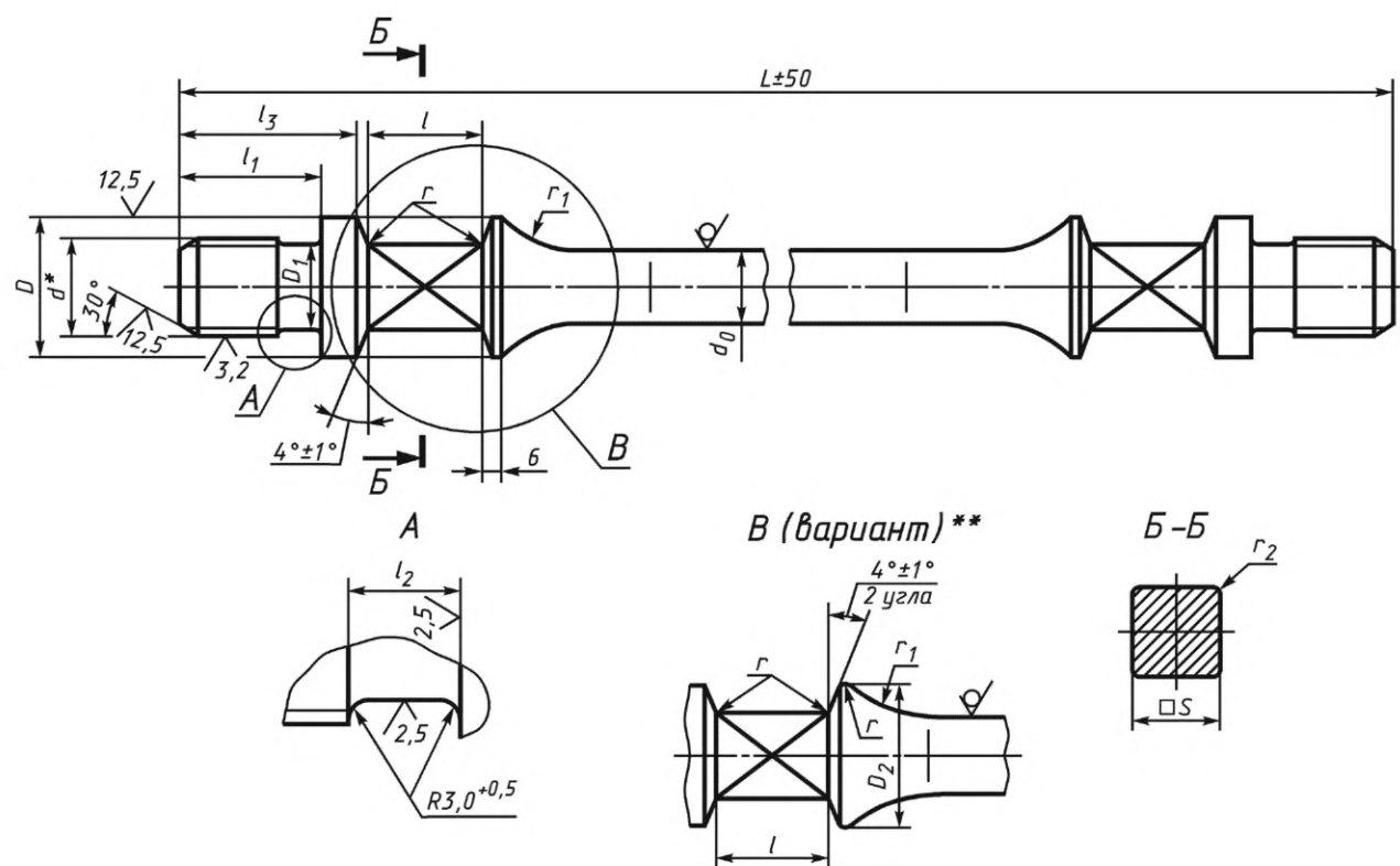
a — металлическая штанга с высаженными головками (ШН)
