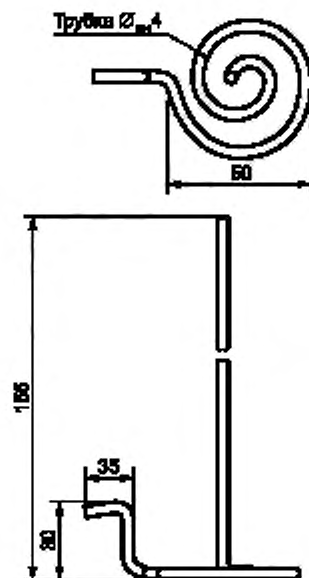
Рисунок 1 — Подающая трубка
