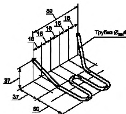
Рисунок 2 — Змеевидная трубка
