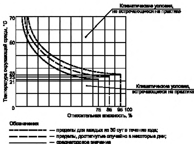
Рисунок А.1 — Соотношение между температурой окружающей среды и относительной влажностью воздуха
