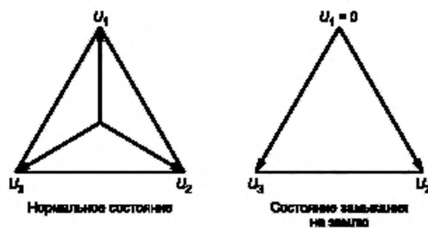
Рисунок С.2 — Напряжения на испытуемом счетчике
