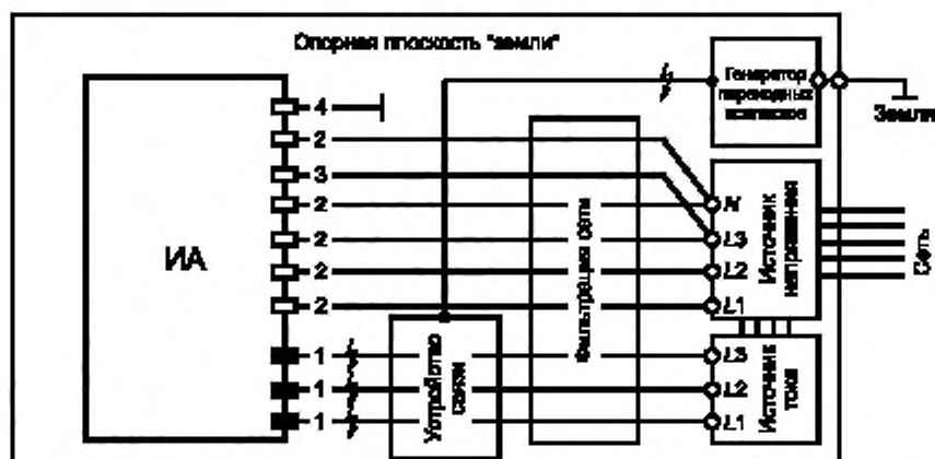
Рисунок Е.3 — Установка для проведения испытаний на устойчивость к наносекундным импульсным помехам. Цели тока
