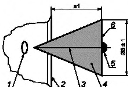
1 — оптическое испытательное выходное устройство; 2 — поверхность счетчика; 3 — оптическая ось датчика; 4 — передаваемый луч; 5 — принимающая головка; 6 — опорная поверхность (оптически активная область, приблизительно 0,5 \text{ см}^2 )
