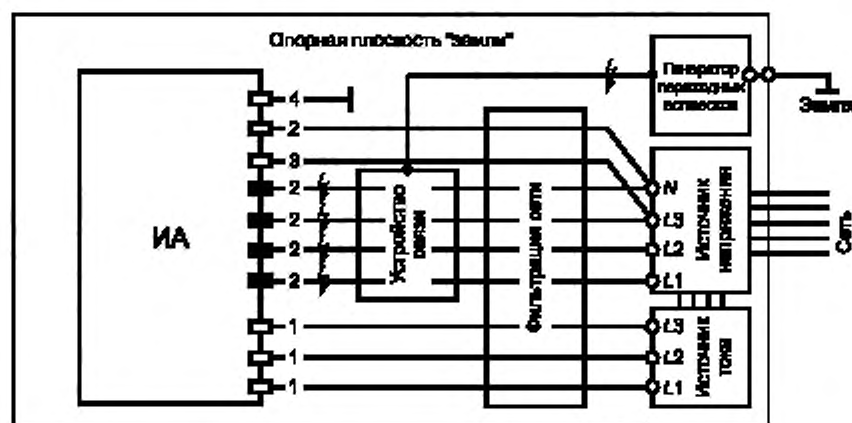
1 — цепи тока; 2 — цепи напряжения; 3 — вспомогательные цепи нормальным напряжением свыше 40 В; 4 — вспомогательные цепи нормальным напряжением до 40 В
