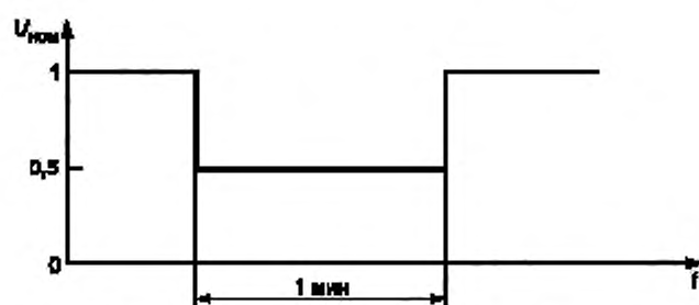
Рисунок В.3 — Провалы напряжения \Delta U = 50\%
