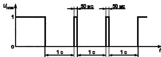
Рисунок В.1 — Прерывания напряжения \Delta U = 100\% , продолжительность 1 с
