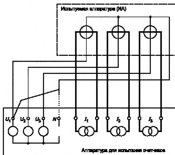
Рисунок С.1 — Схема моделирования состояния замыкания на землю в фазе 1
