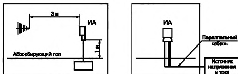
Рисунок Е.1 — Установка для проведения испытаний на устойчивость к электромагнитным радиочастотным полям
