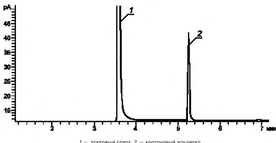
Рисунок 1 — Хроматограмма анализа градуировочной смеси, полученная на хроматографе, оснащенном капиллярной колонкой НР-РРДР*
