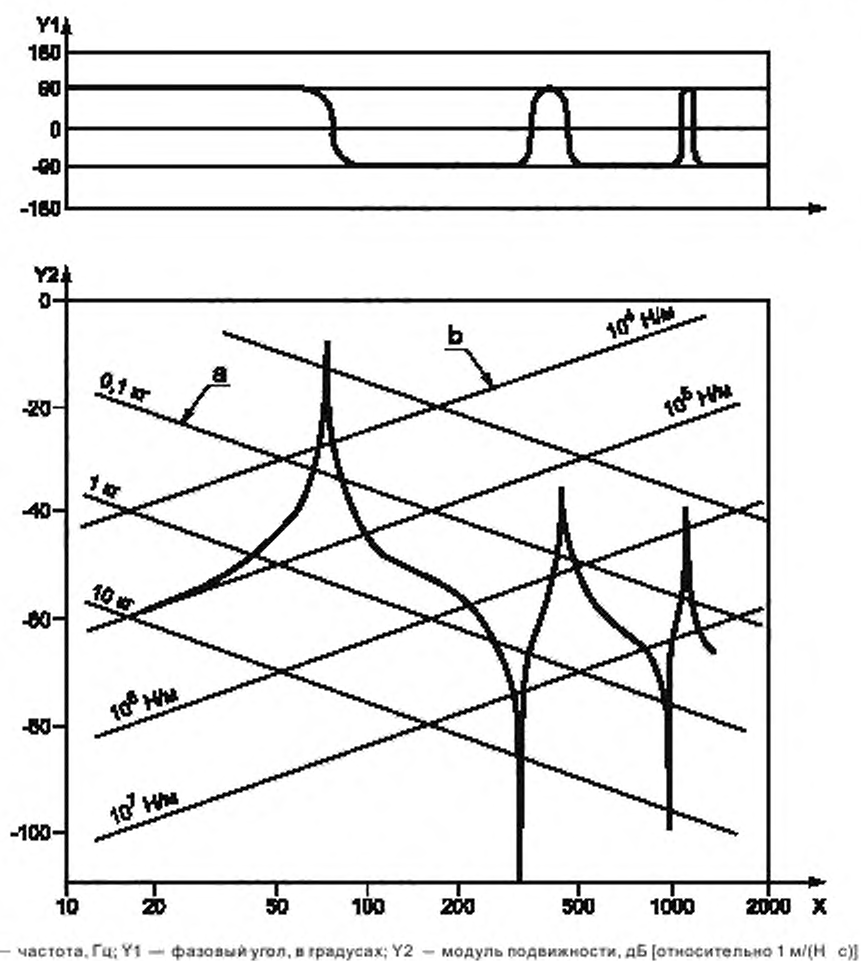
Рисунок 1 — График подвижности
