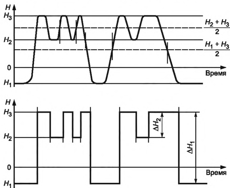
Рисунок 1, лист 1 — Эпюры циклов нагружения
