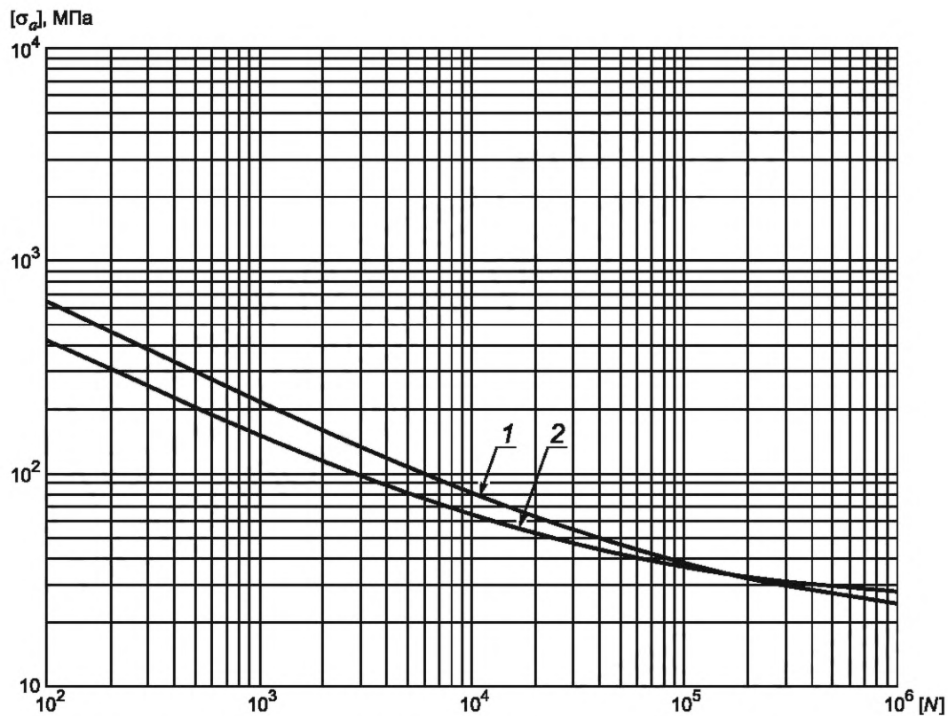
1 — ВТ1-0, ВТ1-00 при A = 0,46 \cdot 10^5 МПа, B = 45,2 МПа, T = 300 °С; 2 — ОТ4-0 при A = 0,33 \cdot 10^5 МПа, B = 58,8 МПа, T = 400 °С
