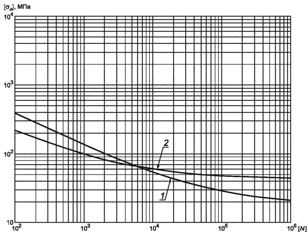
Рисунок 6 — Расчетная кривая усталости для сплавов алюминия
