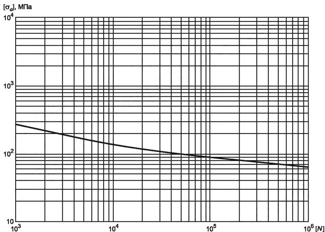
Рисунок 10 — Расчетная кривая усталости для углеродистых и низколегированных сталей с плакировкой из аустенитных сталей (при температуре не более 380 °С)
