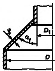
Рисунок 27 — Основные размеры конического перехода
