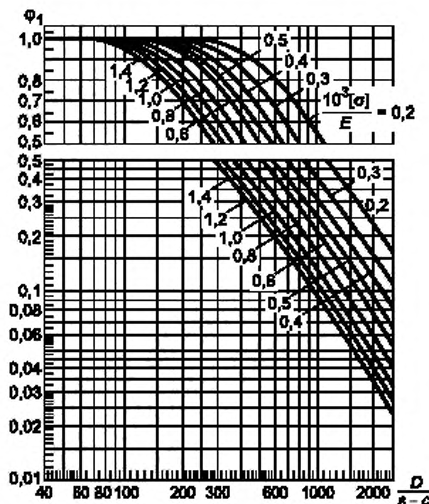
Рисунок 5 — График для определения коэффициента \phi_1
