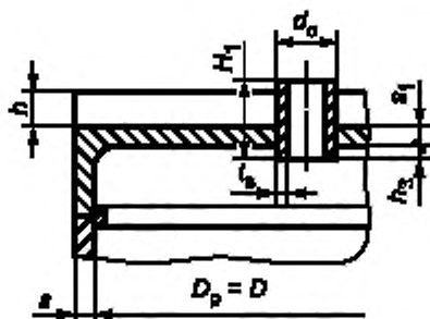
Рисунок 23 — Плоское круглое днище с радиальными ребрами жесткости
