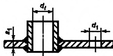
Рисунок 17 — Расчетные размеры отверстий
