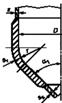
Рисунок 26 — Соединение обечаек с тороидальным переходом
