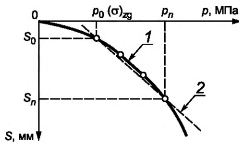
Рисунок Г.1 — График S = f(p) испытания грунта штампом
