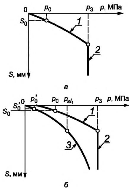
Рисунок Г.1 — График S = f(p) испытания грунта штампом
