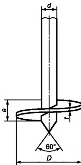
Рисунок Б.1 — Конструкция винтового штампа
