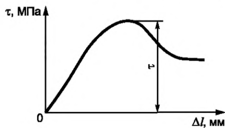
Рисунок А.1 — График \tau = f(\Delta l)
