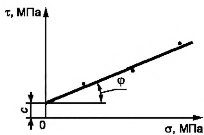
Рисунок А.2 — График \tau = f(\sigma)
