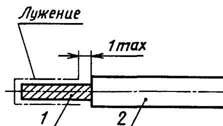
1 — жила; 2 — изоляция
