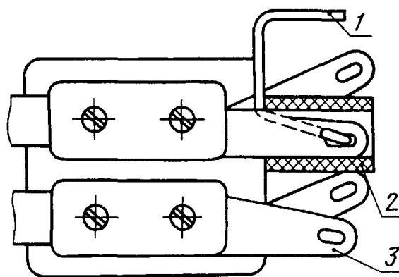
1 — провод; 2 — электроизоляционная трубка на клею; 3 — лепесток
