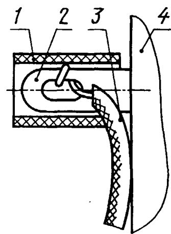
1 — электроизоляционная трубка; 2 — плоский контакт; 3 — провод; 4 — плата
