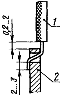
1 — провод; 2 — плоский контакт
