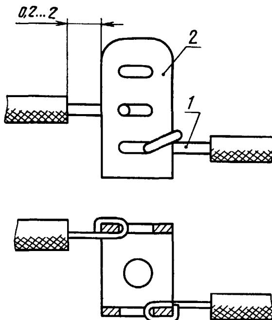
1 — провод; 2 — плоский контакт
