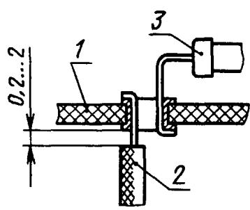
1 — плата; 2 — провод; 3 — элемент
