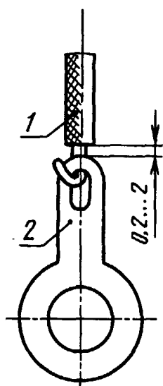
1 — провод; 2 — плоский контакт
