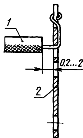
1 — провод; 2 — плоский контакт
