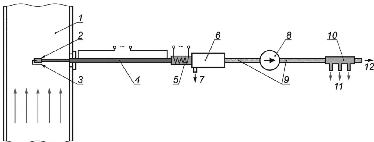
1 — газовод; 2 — фильтр грубой очистки; 3 — защитный металлический щиток; 4 — обогреваемая пробоотборная линия; 5 — обогреваемый фильтр тонкой очистки; 6 — холодильник; 7 — слив конденсата; 8 — побудитель расхода; 9 — необогреваемая пробоотборная линия; 10 — гребенка; 11 — отвод пробы к газоанализаторам; 12 — сброс избыточной газовой пробы
