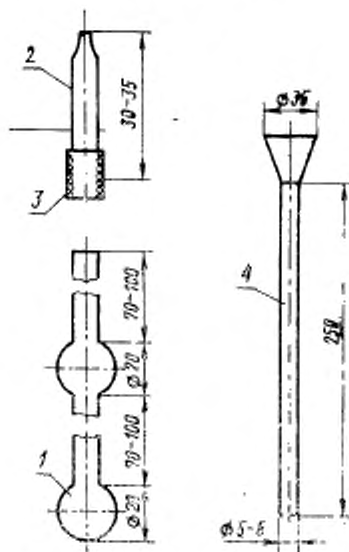
1 — трубка из термостойкого стекла; 2 — стеклянный наконечник с капилляром, 3 — отрезок резиновой трубки; 4 — воронка стеклянная
