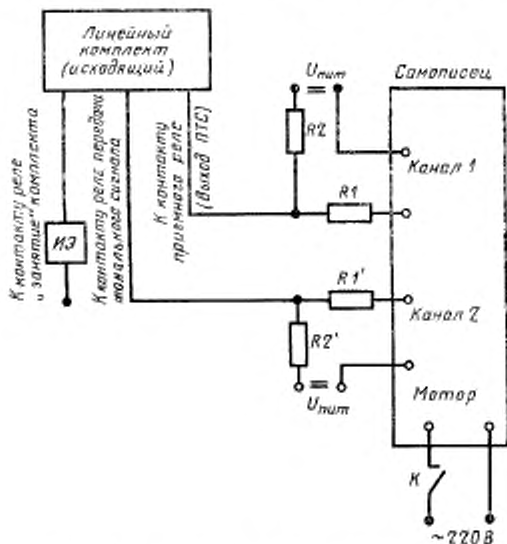
ИЗ — исполнительный элемент, К — контакт исполнительного элемента
