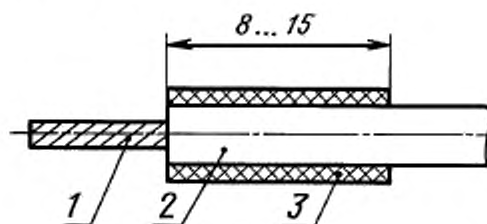
1 — жила; 2 — изоляция; 3 — термоусаживаемая трубка
