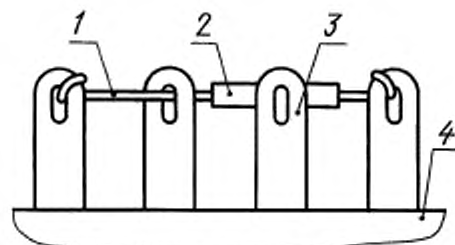
1 — провод; 2 — электроизоляционная трубка; 3 — плоская контакт-деталь; 4 — плата
