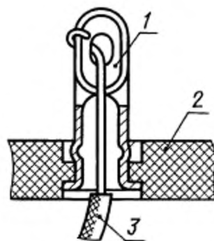
1 — плоская контакт-деталь; 2 — плата; 3 — провод
