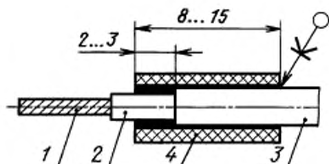
1 — жила; 2 — изоляция; 3 — защитный покров; 4 — электроизоляционная трубка
