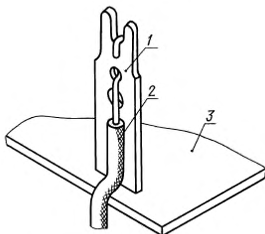
1 — плоская контакт-деталь; 2 — провод; 3 — плата
