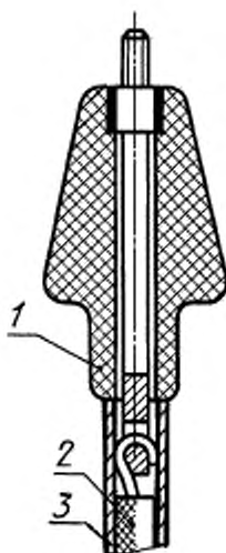
1 — изолятор; 2 — провод; 3 — электроизоляционная трубка
