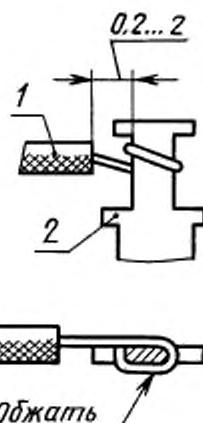
1 — провод; 2 — плоская контакт-деталь
