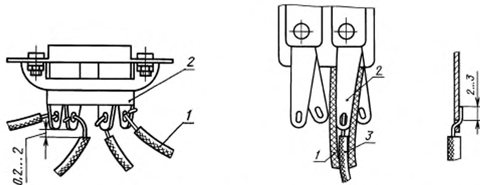
1 — электроизоляционная трубка на клею; 2 — лепесток; 3 — провод
