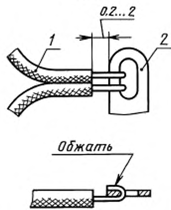
1 — провод; 2 — плоская контакт-деталь
