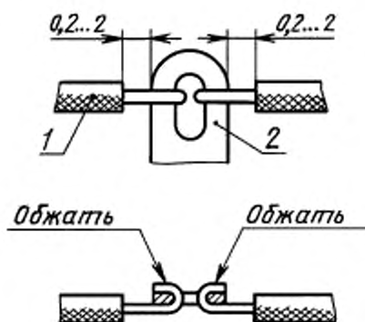
1 — провод; 2 — плоская контакт-деталь
