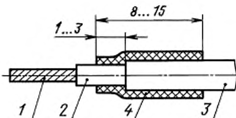
1 — жила; 2 — изоляция; 3 — защитный покров; 4 — термоусаживаемая трубка
