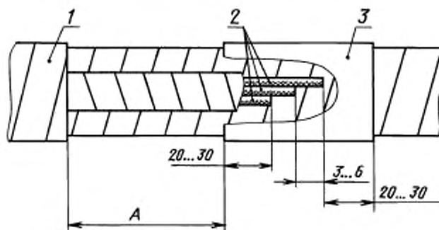
1 — жгут; 2 — запасные провода; 3 — бандаж из электроизоляционного материала
