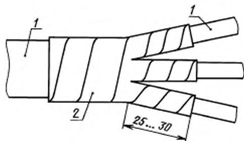
1 — электроизоляционная трубка; 2 — электроизоляционная лента
