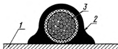
1 — панель; 2 — компаунд; 3 — жгут
