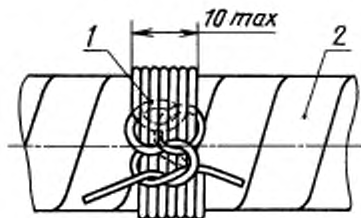
1 — бандаж из ниток; 2 — жгут
