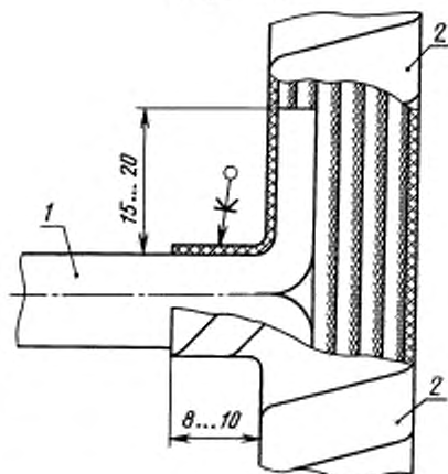
1 — электроизоляционная трубка; 2 — электроизоляционная лента
