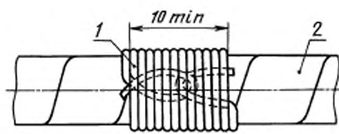
1 — бандаж из ниток; 2 — жгут
