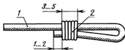
1 — провод; 2 — бандаж из ниток
