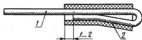
1 — провод; 2 — электроизоляционная трубка
