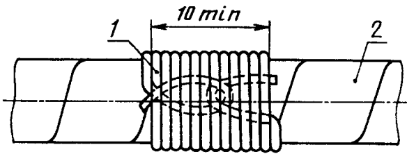
1 — бандаж из ниток; 2 — жгут
