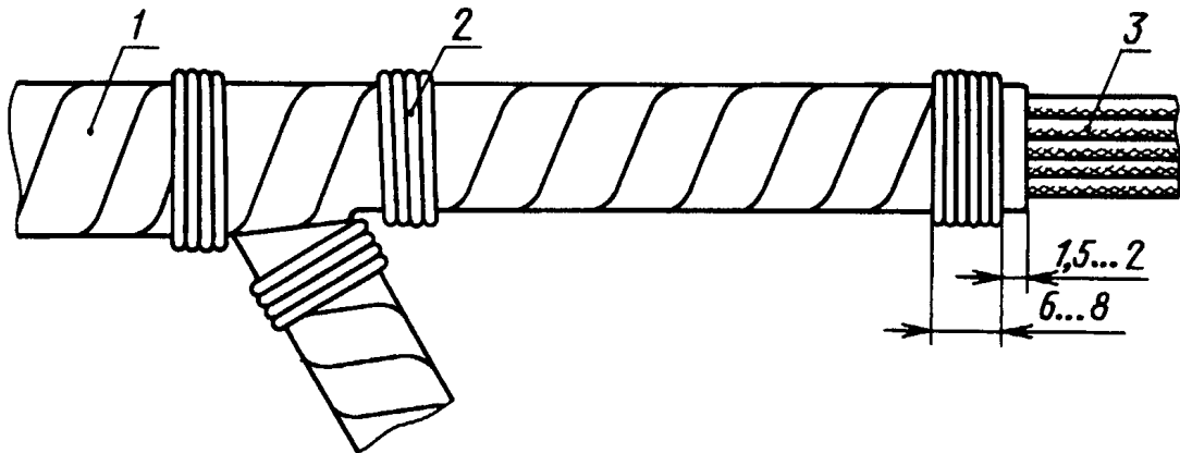
1 — электроизоляционная лента; 2 — бандаж из ниток; 3 — жгут
