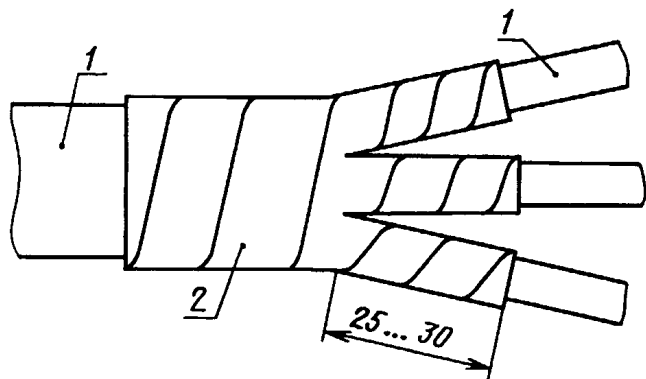
1 — электроизоляционная трубка; 2 — электроизоляционная лента.
