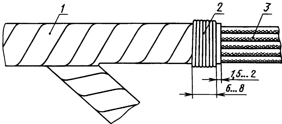
1 — электроизоляционная лента; 2 — бандаж из ниток; 3 — жгут
