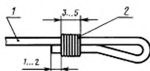
1 — провод; 2 — нитяной бандаж
