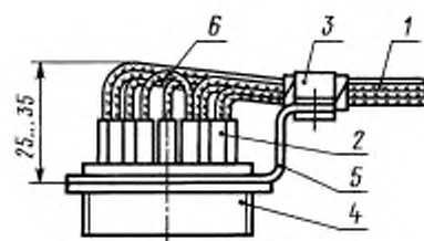
1 — жгут; 2 — нитяной бандаж (скоба); 3 — изоляционные трубки; 4 — соединитель; 5 — кронштейн; 6 — перемычка
