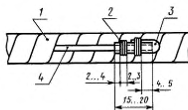
1 — жгут; 2 — нитяной бандаж; 3 — изоляционная трубка; 4 — провод
