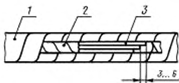
1 — жгут; 2 — изоляционная лента; 3 — резервные провода
