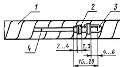
1 — жгут; 2 — нитяной бандаж; 3 — изоляционная трубка; 4 — провод
