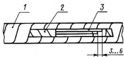
1 — жгут; 2 — изоляционная лента; 3 — резервные провода
