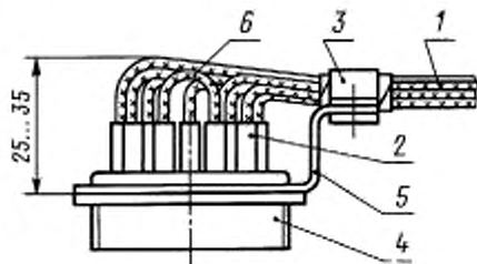
1 — жгут; 2 — изоляционная трубка; 3 — скоба; 4 — соединитель; 5 — кронштейн; 6 — перемишка
