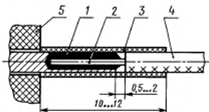
1 — припой; 2 — жила; 3 — изоляционная трубка; 4 — провод; 5 — соединитель
