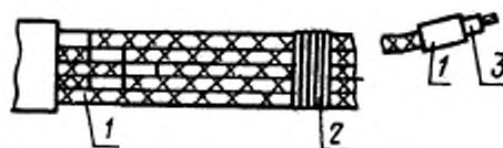
1 — бирки; 2 — бандаж; 3 — наконечник
