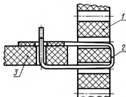
1 — гибкая матрица; 2 — хомут; 3 — ячейка
