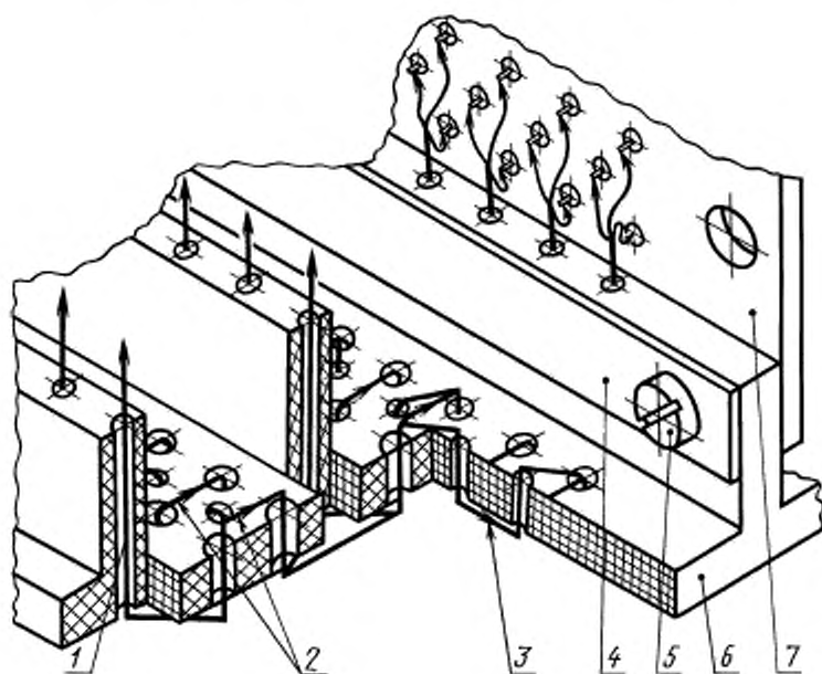
Пример прошивки гибкой матрицы монтажными проводами
