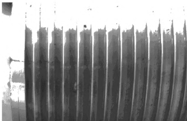
Рисунок 17 — Трещина на заходной фаске и наружной резьбе
