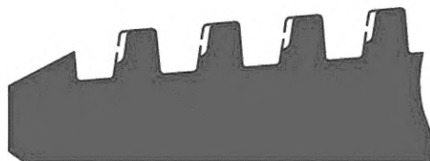
б) Подрез боковой стороны и резьбы вершины витка резьбы
