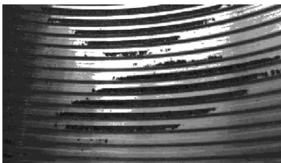
б) Черновины по части поверхности витков внутренней резьбы
