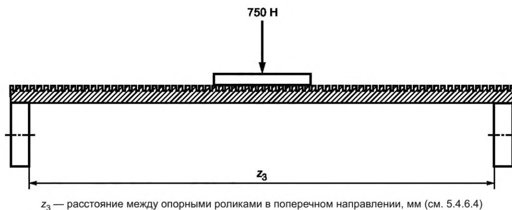
Рисунок 8 — Лента (вид в разрезе), одиночное усилие
