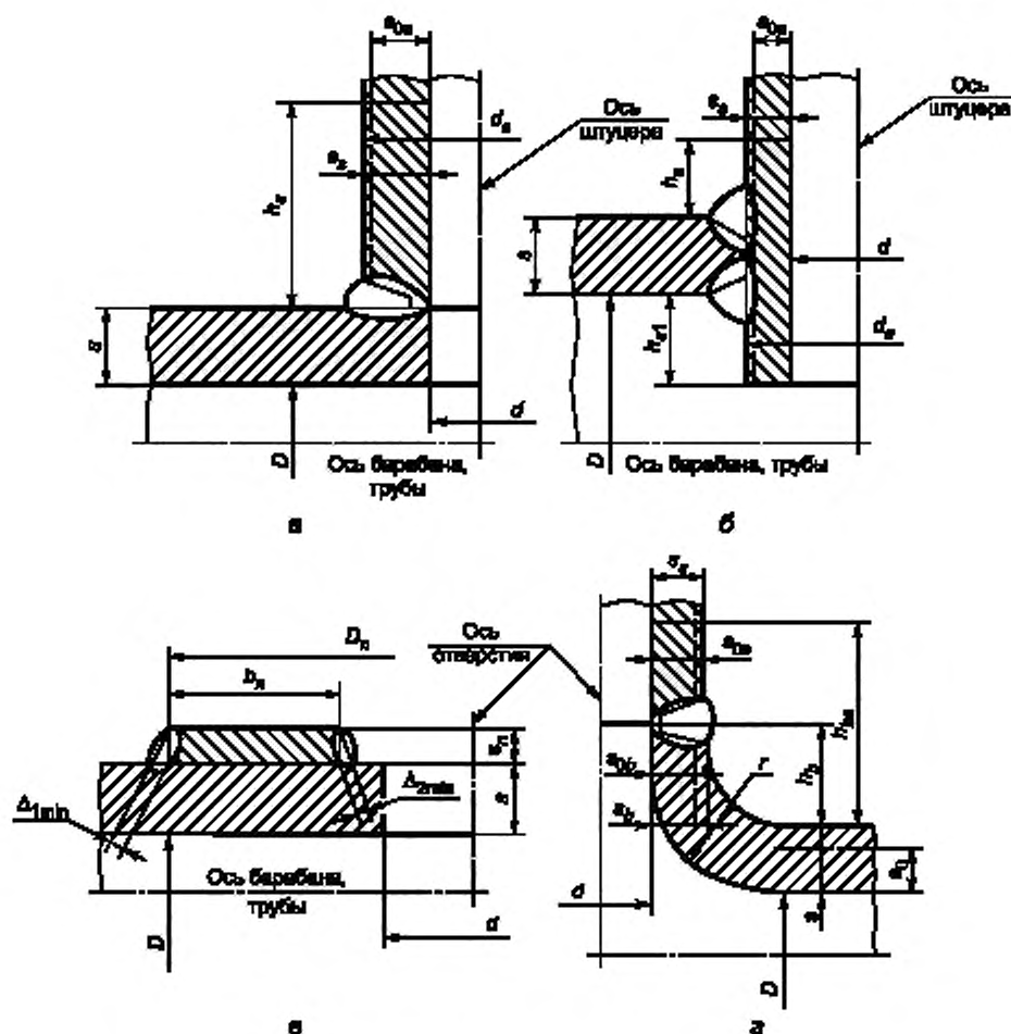
а — укрепление наружным штуцером, б — укрепление проходным штуцером; в — укрепление накладкой; г — укрепление вытянутой горловиной; s_{об} = s_{ос} при одинаковой марке стали
