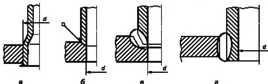
а — отверстие с завальцованной трубой (штуцером); б — отверстие с приварным штуцером (трубой) без полного проплавления толщины стенки штуцера (конструктивный зазор); в — отверстие с приварным штуцером (трубой) при полном проплавлении толщины стенки штуцера; г — отверстие с приварным штуцером (трубой) при полном проплавлении толщины стенки расчетной детали
