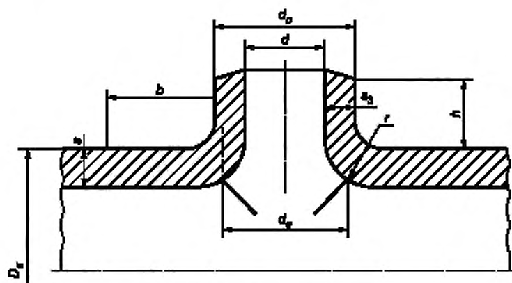
Рисунок 13 — Вытянутая горловина
