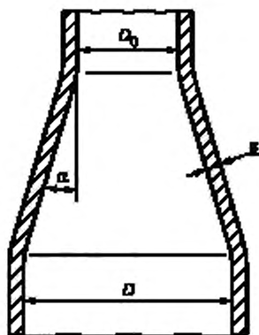
Рисунок 1 — Схема конического переходного участка
