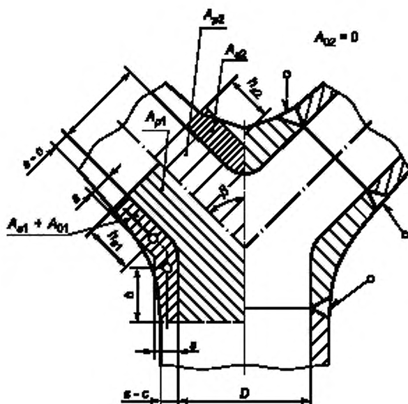
Рисунок 24 — Схема развилки
