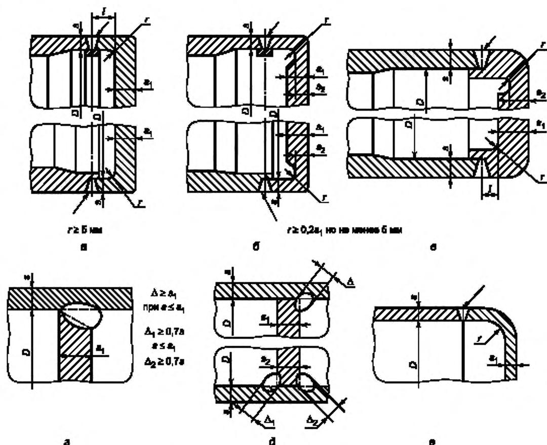
Рисунок 4 — Типы плоских донн
