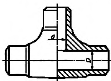
Рисунок 22 — Схема ковкого тройника
