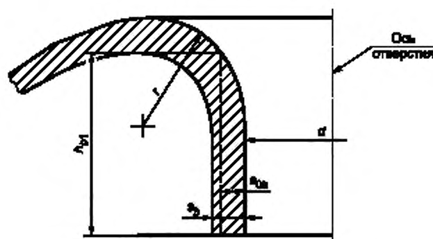
Рисунок 14 — Отбортованный воротник
