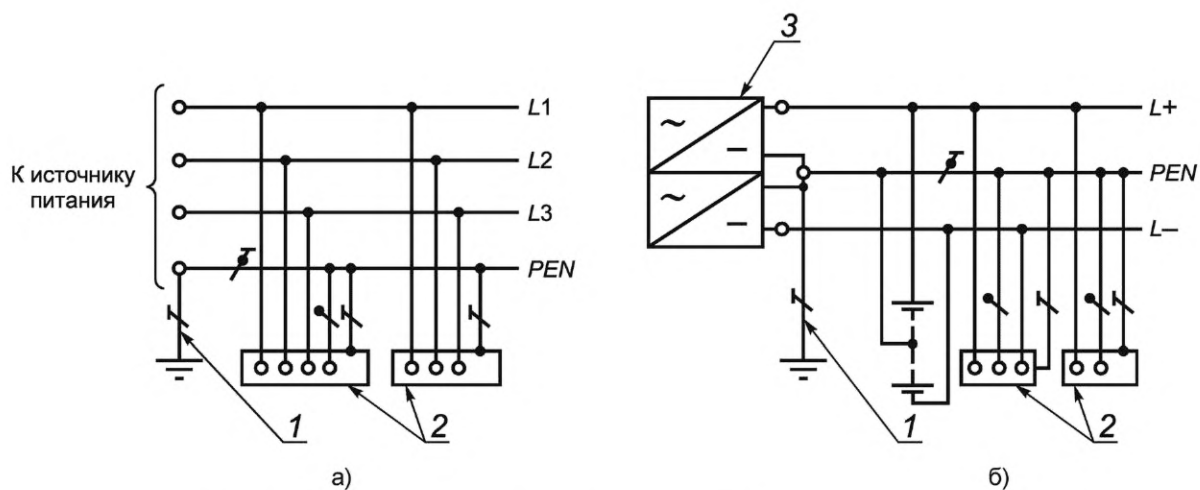
Рисунок 21 — Система TN-C переменного (а) и постоянного (б) тока. Нулевой защитный и нулевой рабочий проводники совмещены в одном проводнике
