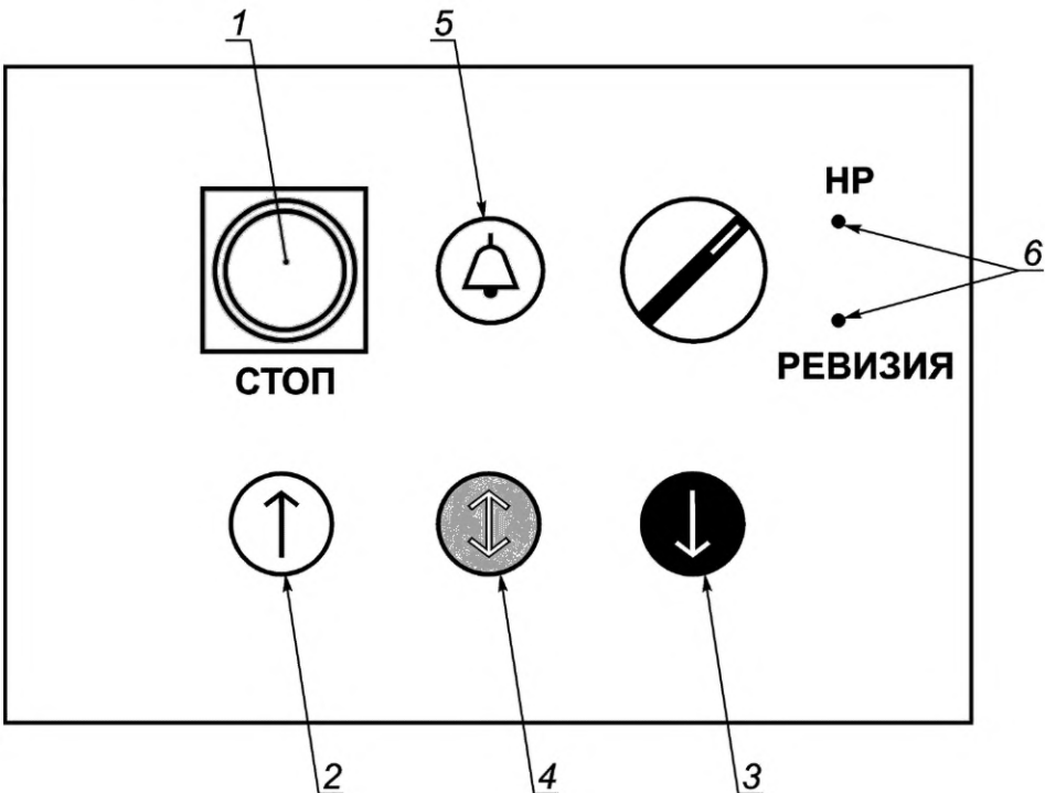
1 — кнопка «Стоп»; 2 — кнопка движения вверх; 3 — кнопка движения вниз; 4 — кнопка ход; 5 — кнопка экстренной сигнализации; 6 — переключатель режима работы
