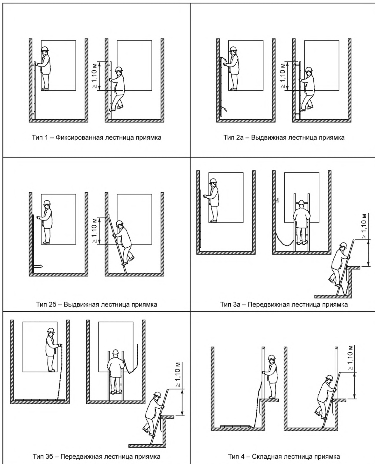
Рисунок В.1 — Типы лестниц доступа в приямок
