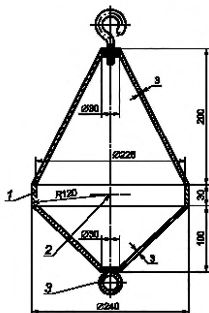
1 — ударное кольцо; 2 — базисная точка для измерения высоты падения; 3 — крепление пускающего приспособления
