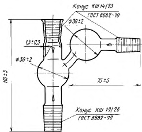
Каплеуловитель
