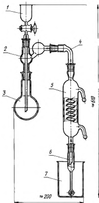
Прибор для отделения мышьяка в сталях, чугунах и сплавах
