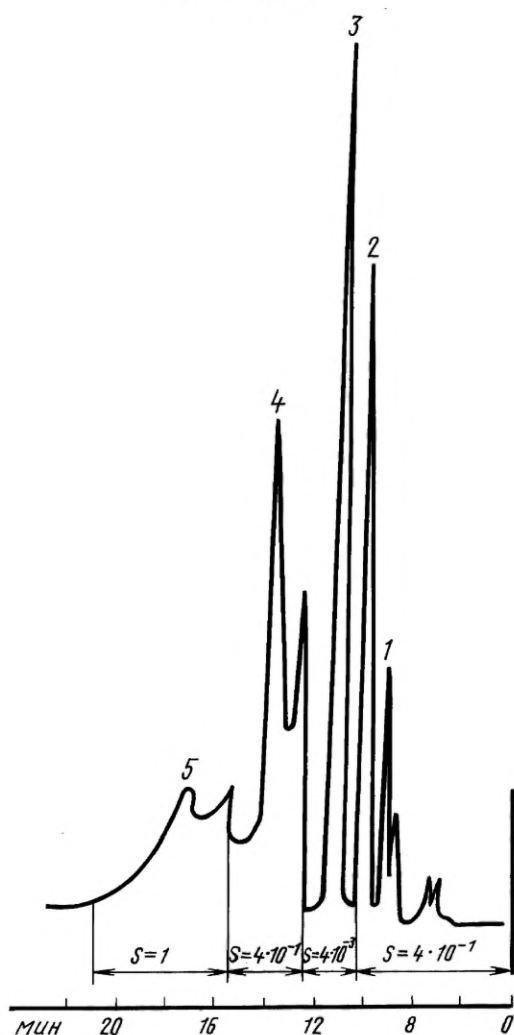
Хроматограмма
