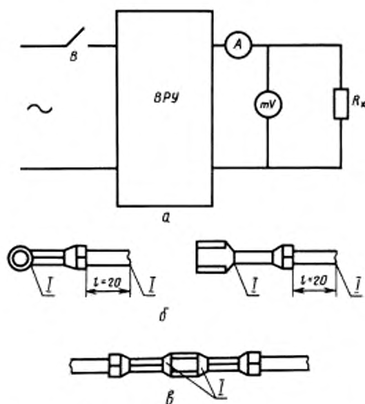
Схема измерения падения напряжения
