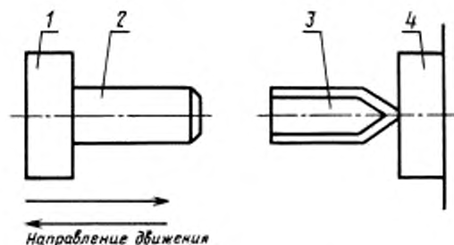
Схема приспособления для измерения усилия соединения и разъединения штекерных наконечников
