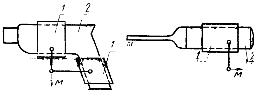
а б 1—металлическая фольга; 2—корпус из изоляционного материала; М—точка присоединения эквивалента руки
