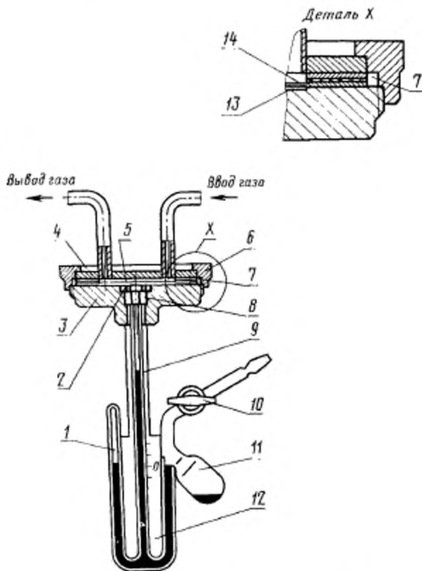
1 - U-образная трубка; 2 - перфорированный диск; 3 - нижняя часть камеры; 4 - верхняя часть камеры; 5 - рабочий объем верхней части камеры; 6 - запирающее устройство; 7 - резиновая прокладка; 8 - уплотнение; 9 - калиброванная трубка; 10 - запорный кран; 11 - резервуар с ртутью; 12 - шкала с ценой деления 0,5 мм; 13 - фильтровальная бумага; 14 - испытываемый образец.
