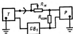
Т—телеграфный аппарат; ГБ_1 —линейная батарея; R_N —сопротивление нагрузки; R_{изм} —измерительное сопротивление; P —измерительный прибор
