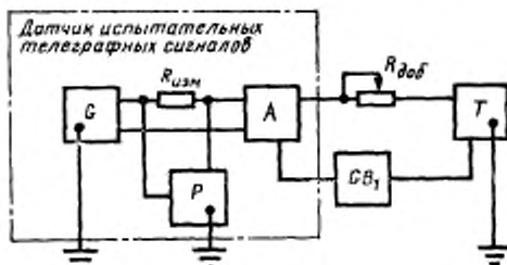
G—генератор прямоугольных импульсов; R_{изм} —измерительное сопротивление; P—измеритель временных интервалов; A—выходное реле; GB 1 —линейная батарея; R_{доб} —добавочное сопротивление; T—телеграфный аппарат
