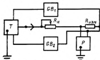
Т—телеграфный аппарат; ГБ_1 , ГБ_2 —линейные батареи; R_N —сопротивление нагрузки; R_{изм} —измерительное сопротивление; P —измерительный прибор
