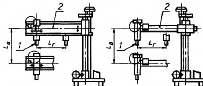
Для самоходного сварочного автомата Для подвесного сварочного автомата
