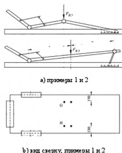
Рисунок В.3 — Испытания сиденья на долговечность
