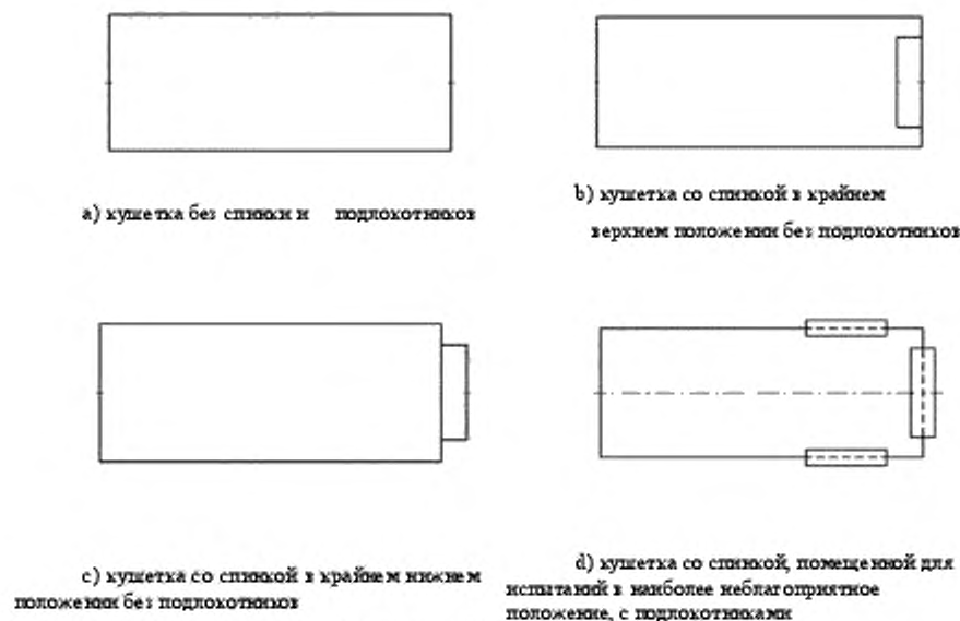
Рисунок В.1 — Виды кушеток
