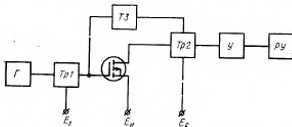
\Gamma — генератор; Tr1 — входной трансформатор полного сопротивления; Tr2 — выходной трансформатор полного сопротивления; T3 — схема нейтрализации; Y — усилитель; RУ — регистрирующее устройство.
