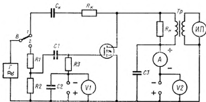
\Gamma —генератор; R_1 , R_2 , R_3 , R_n , R_K —резисторы; C_1 , C_2 , C_3 , C_K —конденсаторы; Tр —трансформатор; A —измеритель тока; V_1 , V_2 , ИП —измерители напряжения; B —переключатель
