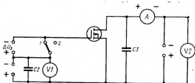
C2, C3 —конденсаторы; V1, V2 —измерители напряжения; A —измеритель тока; \Delta U_x —источник постоянного напряжения.
