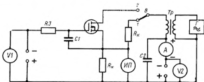
Г—генератор; R3, RN, RK—резисторы; C1, C2—конденсаторы; V1, V2, ИП—измерители напряжения; А—измеритель тока; Tr—трансформатор; В—переключатель.
