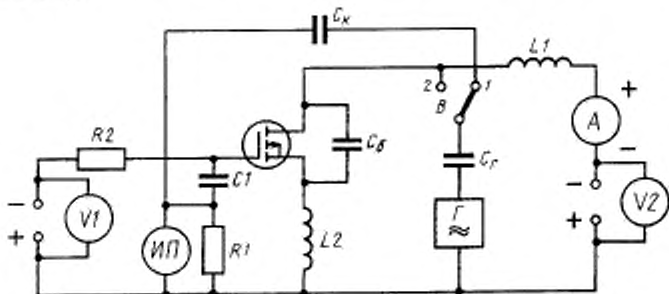
Г—генератор; R_1 , R_2 —резисторы; C_1 , C_x , C_0 , C_g —конденсаторы; L_1 , L_2 —дроссели; V_1 , V_2 , ИП—измерители напряжения; А—измеритель тока; В—переключатель.
