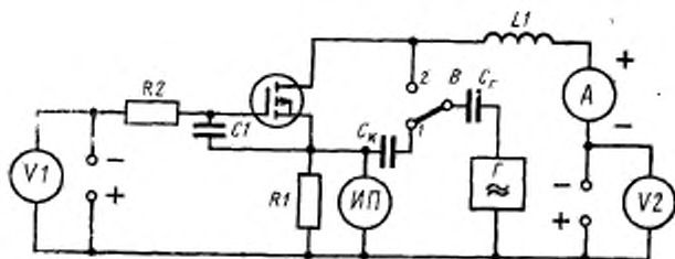
Г—генератор; R_1 , R_2 —резисторы; C_1 , C_k , C_g —конденсаторы; L_1 —дроссель; V_1 , V_2 , ИП—измерители напряжения; А—измеритель тока; В—переключатель.
