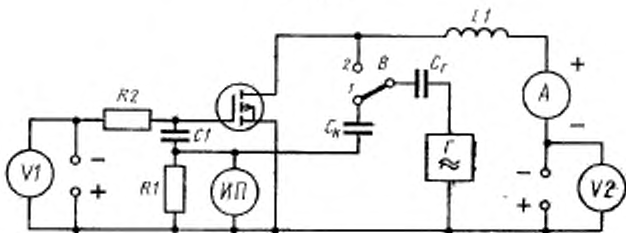
Г—генератор; R_1 , R_2 —резисторы; C_1 , C_x , C_0 , C_g —конденсаторы; L_1 —дроссель; V_1 , V_2 , ИП—измерители напряжения; А—измеритель тока; В—переключатель.
