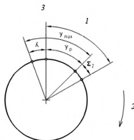
1 – максимальный перебег ( =\gamma_p + \varepsilon_1 ); 2 – направление вращения, 3 – OU; \lambda – смещение положения останова
