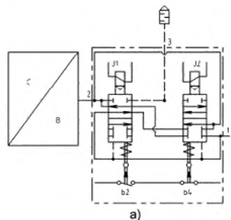
а) Выход клапана без давления
