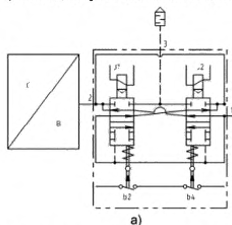
а) Выход второго клапана под давлением
