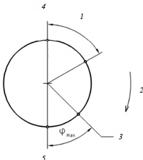
1 – максимальный перебег ( = \gamma_p + \varepsilon ); 2 – направление вращения; 3 – точка начала прерывания действия/глушения; 4 – ОУ; 5 – УУ
