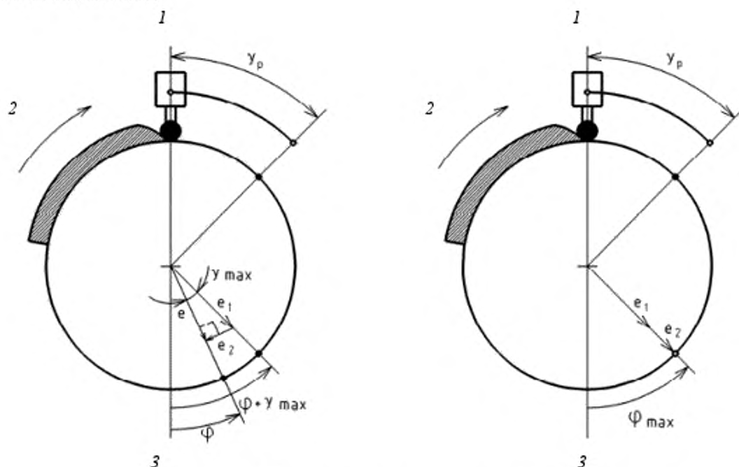
1 — ОУ; 2 — направление вращения; 3 — УУ
