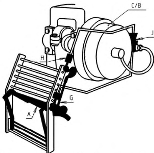
Рисунок А.1 – Пример блокировочного ограждения с резервированием и самоконтролем [см. перечисление b) А.1.1]
