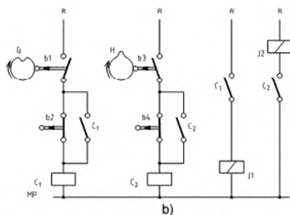
б) Ограждение открыто
