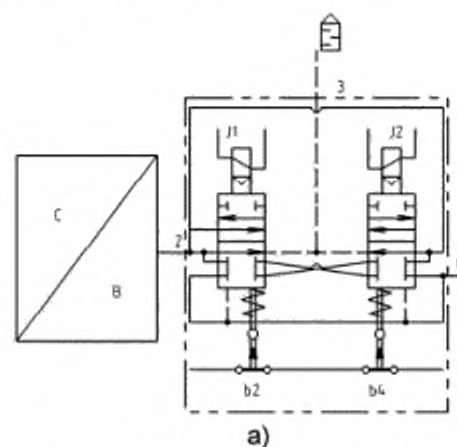
а) Выход второго клапана без давления
