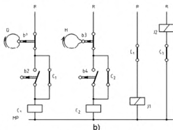
б) Ограждение закрыто (цикл включен)
